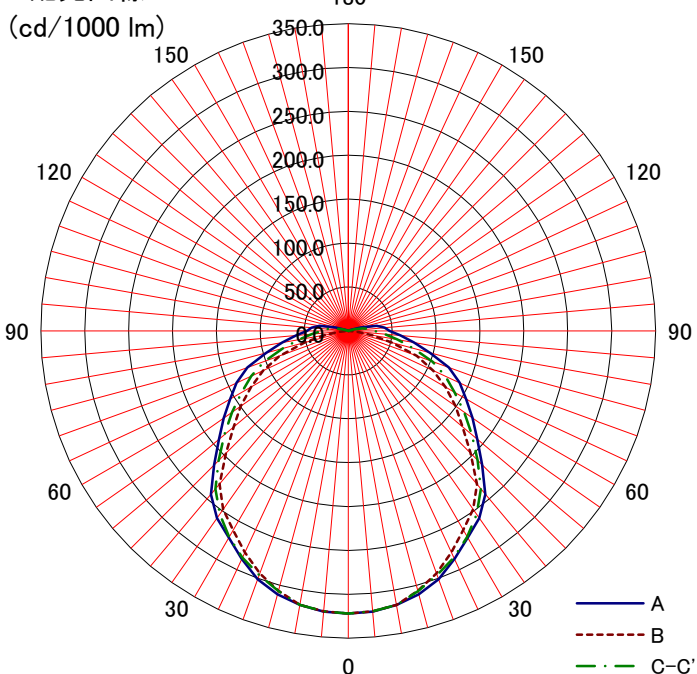
配光曲線
